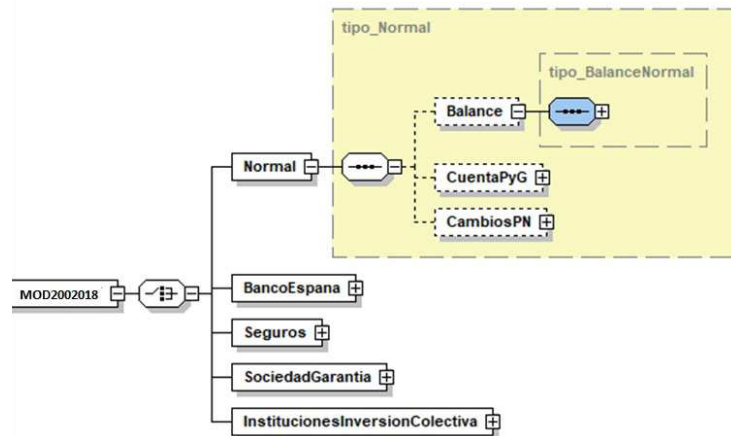
Esquema mod2002018.xsd
