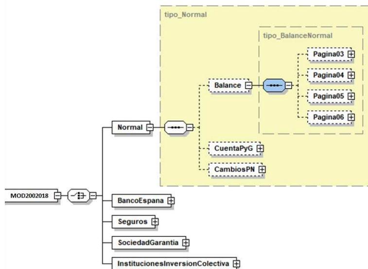
Esquema mod2002018.xsd
